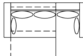
B-337/Gr - GARNITURA S KRAĆOM DAMSKOM 243x160x75 cm LEŽAJ 200x147 cm SPREMIŠTE ZA POSTELJINU 2-58x65x15 cm
